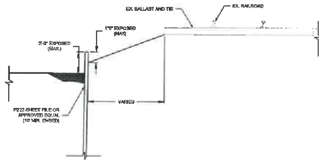
SHEET PILE DETAIL 3 N.T.S.
